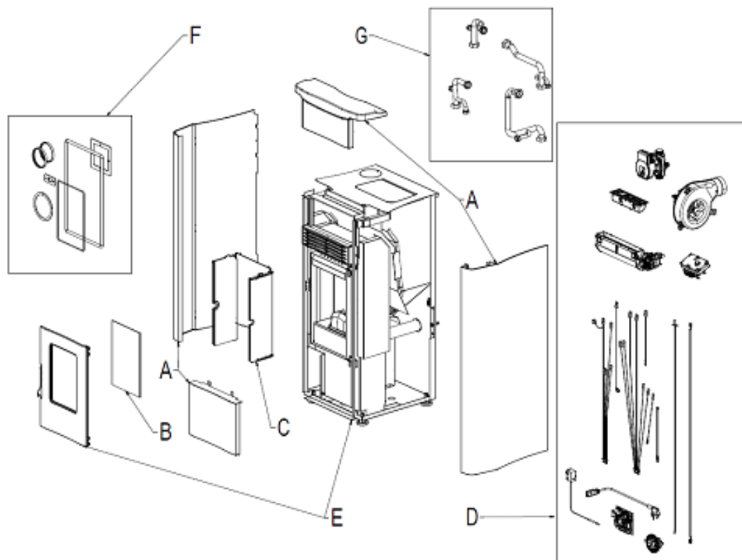
Fig. 1 - Explosionszeichnung
