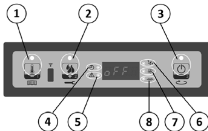
Fig. 6 - Display: Leds eingeschaltet
