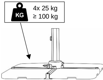
Abb. 3-2 Aufstellen des Plattenständers
