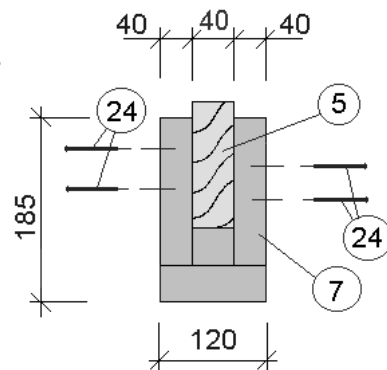
Schnitt A - A
