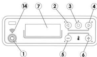
Fig. 9 - Bedientafel (wi-fi)
