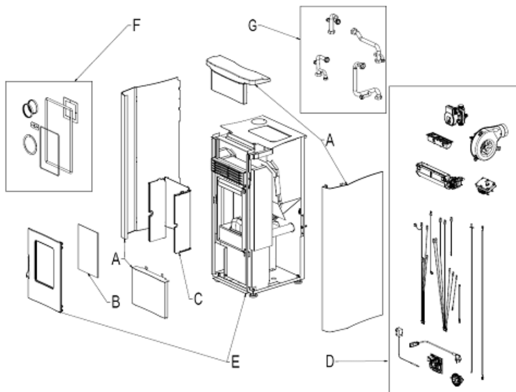
Fig. 1 - Explosionszeichnung
