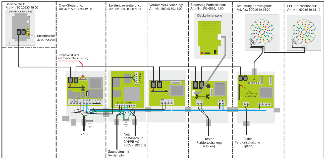
Abbildung 4 Anschlussbeispiel Ofensteuerung
