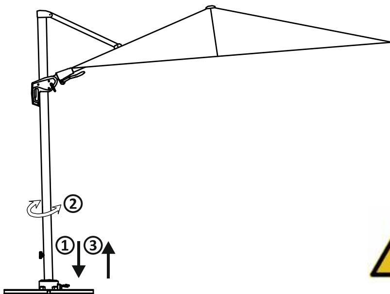
Abb. 4-3 Drehen des Schirms
