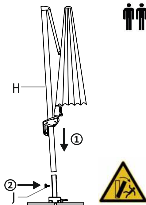
Abb. 3-3 Aufstellen des Schirms
