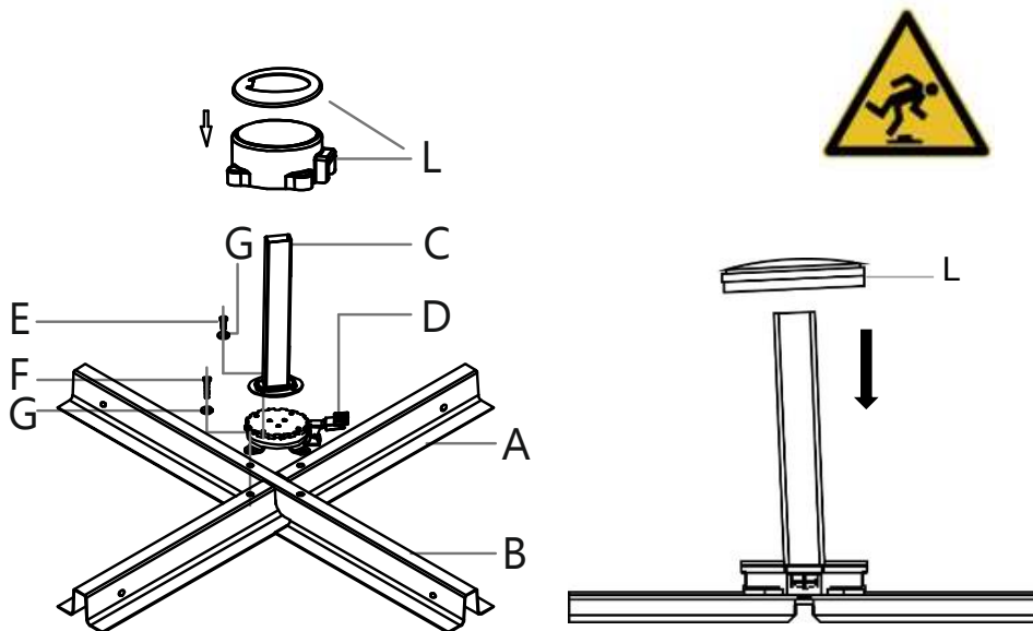
Abb. 3-1 Montage des Plattenständers
