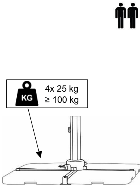
Abb. 3-2 Aufstellen des Plattenständers
