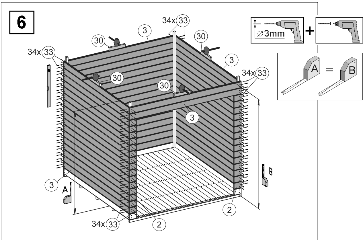
Abbildung Art.-Nr.: 227.2121.10400
