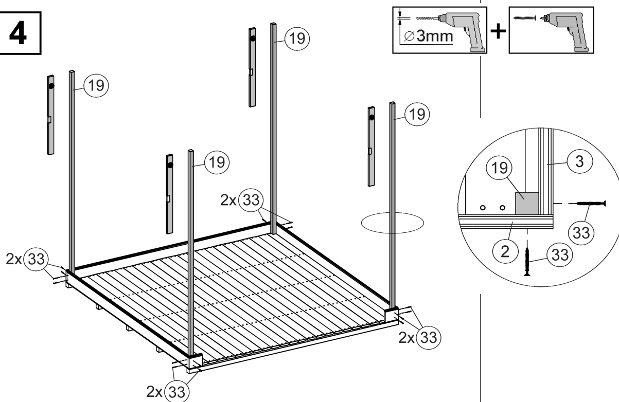
Abbildung Art.-Nr.: 227.2121.10400
