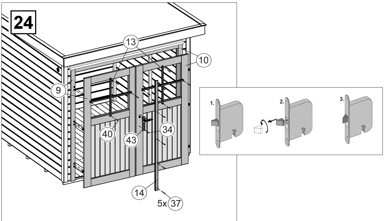
Abbildung Art.-Nr.: 227.2121.10400
