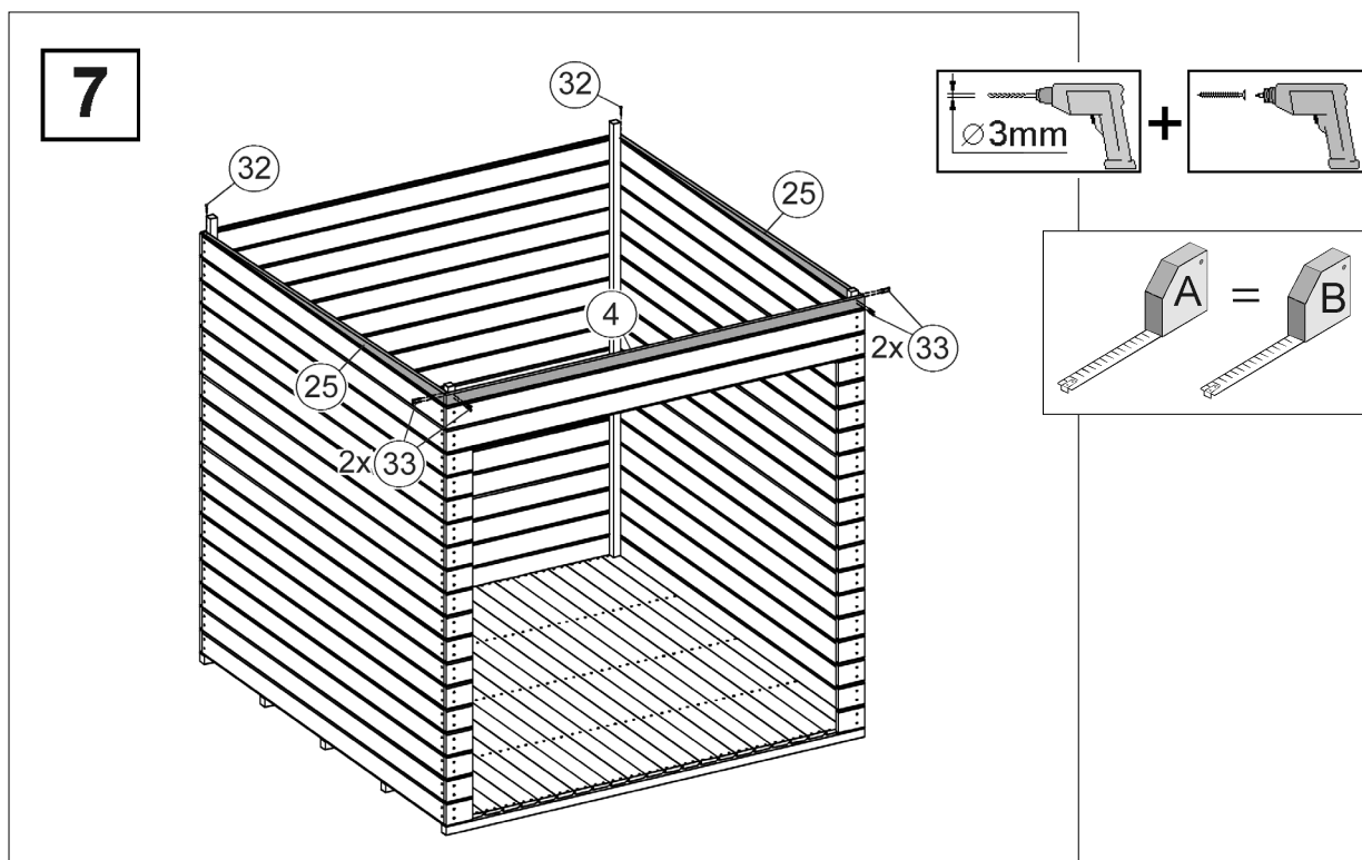
Abbildung Art.-Nr.: 227.2121.10400
