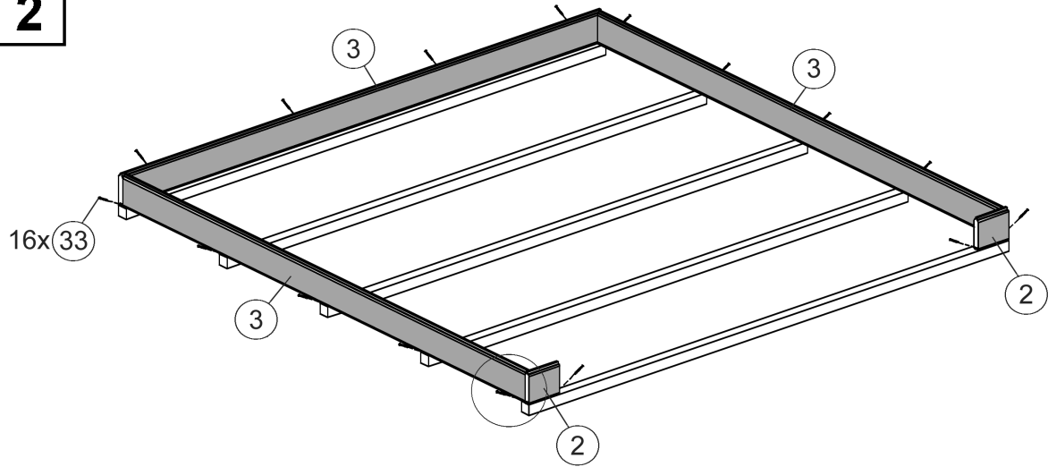
Abbildung Art.-Nr.: 227.2121.10400
