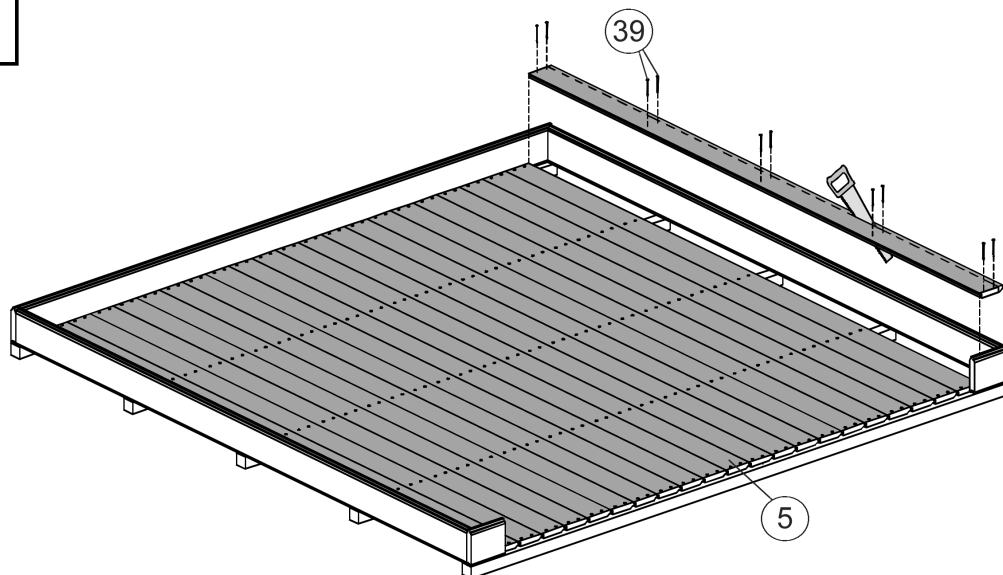
Abbildung Art.-Nr.: 227.2121.10400
