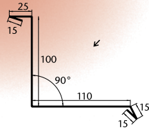
Unteres Traufblech / Rinneneinlaufblech
