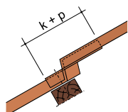
Verbindung der Tafeln am Querfals
