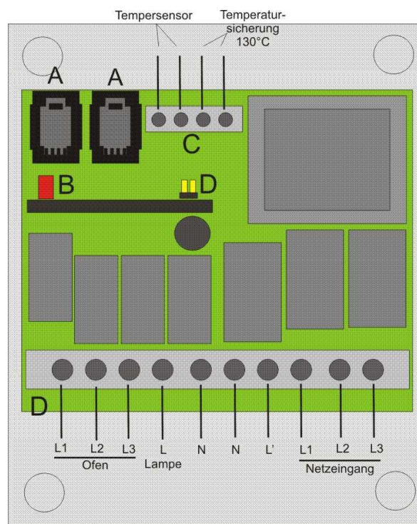
Abbildung 1 Anschlüsse
