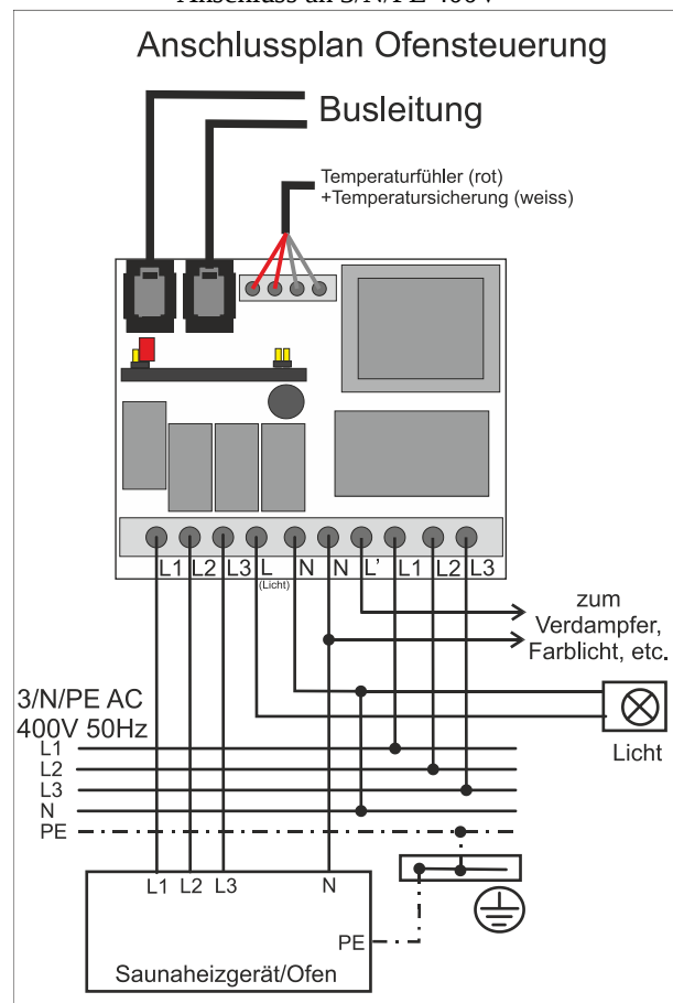
Abbildung 7 Anschlussplan 400V
