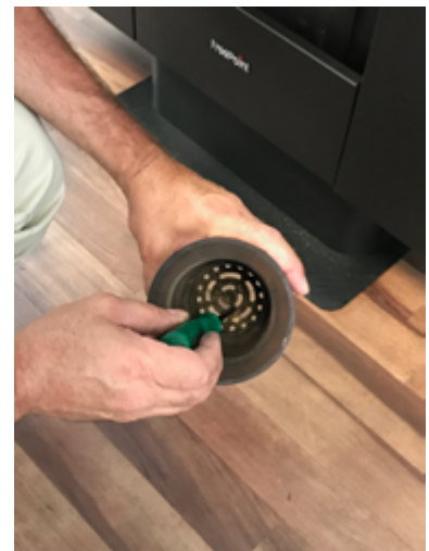
Fig. 37 - Reinigung Brennschale
