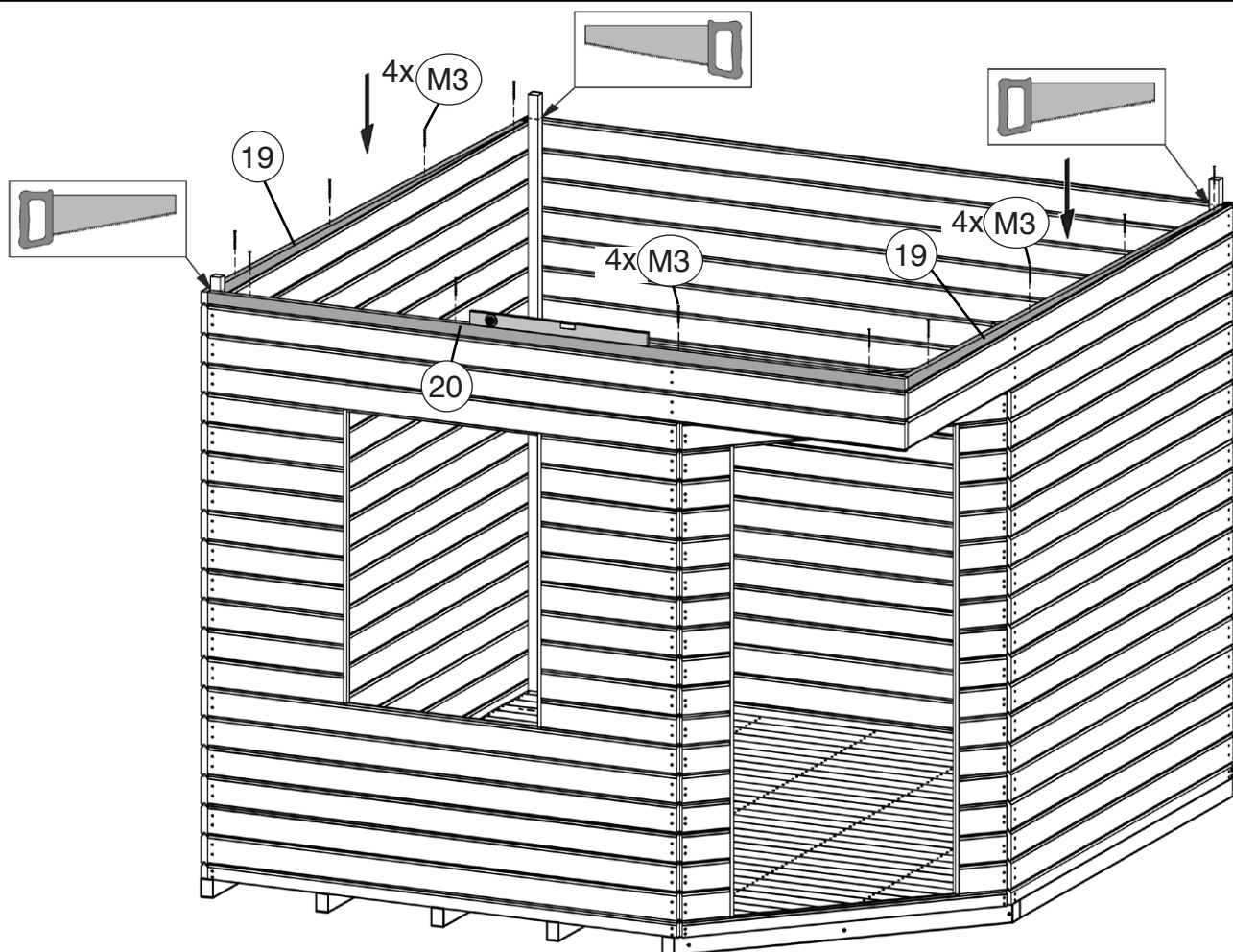
Abb.: Ausrichtung des Gefälles, Richtung des Gefälles durch die Anordnung der oberen Abschlussbohlen variabel! Bei der zusätzlichen Montage eines Anbaus Richtung des Gefälles des Anbaus beachten! (siehe Grafik oben)
