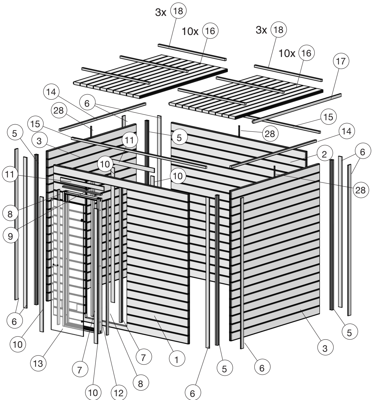
Abb.: VARIA 1
