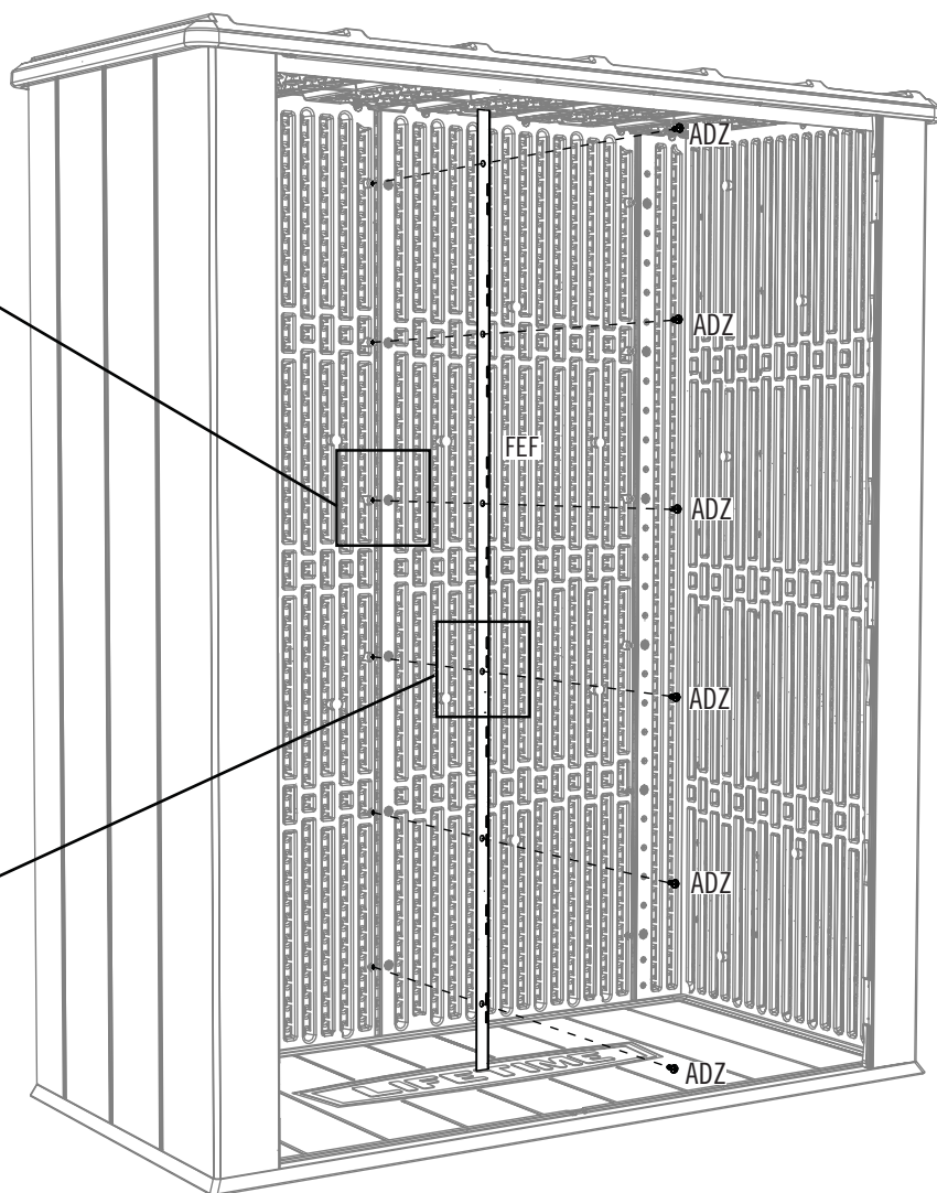
Fessure sul bordo destro del canale / Schlitze auf der rechten Kante des Profils / Прорези на правом краю швеллера
