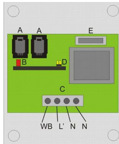
Abbildung 1 Anschlüsse
