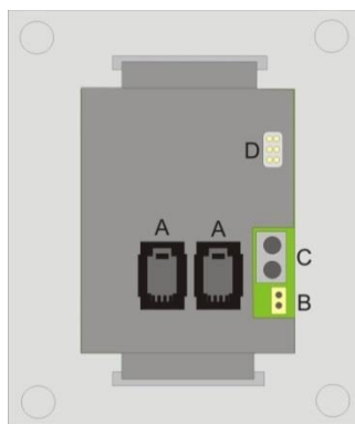
Abbildung 2 Ansicht hinten BDE
